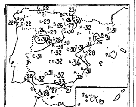
Temperaturas máximas del día 2
