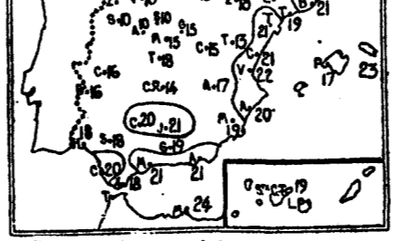
Temperaturas mínimas del día 2
