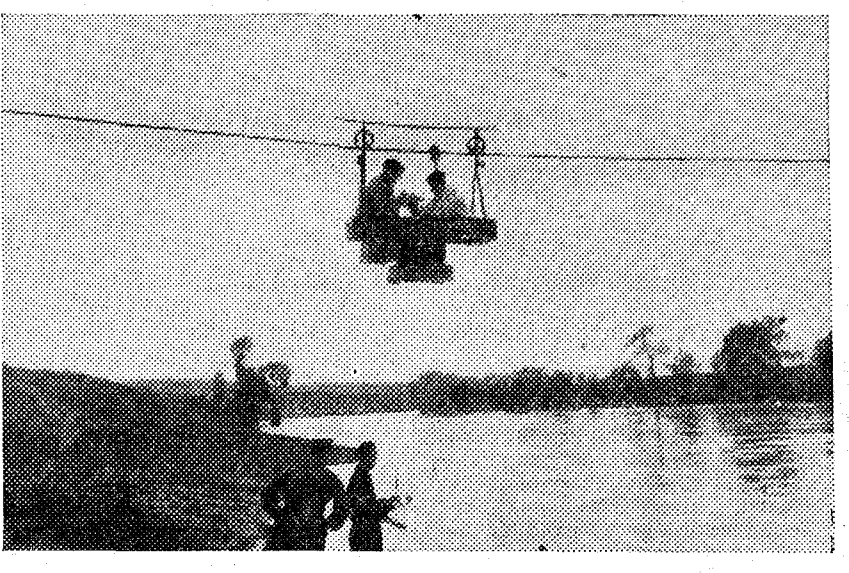
Sistema de aforos en la estación de Portusa
