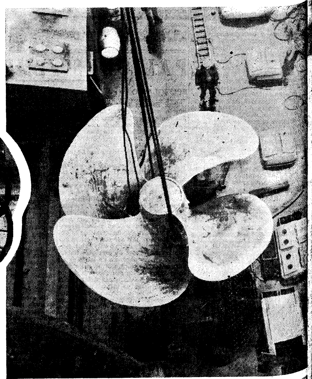
La nueva hélice construída para el «Normandie» mide cinco metros y medio de diámetro, y pesa 28 toneladas (Foto Vidal)
