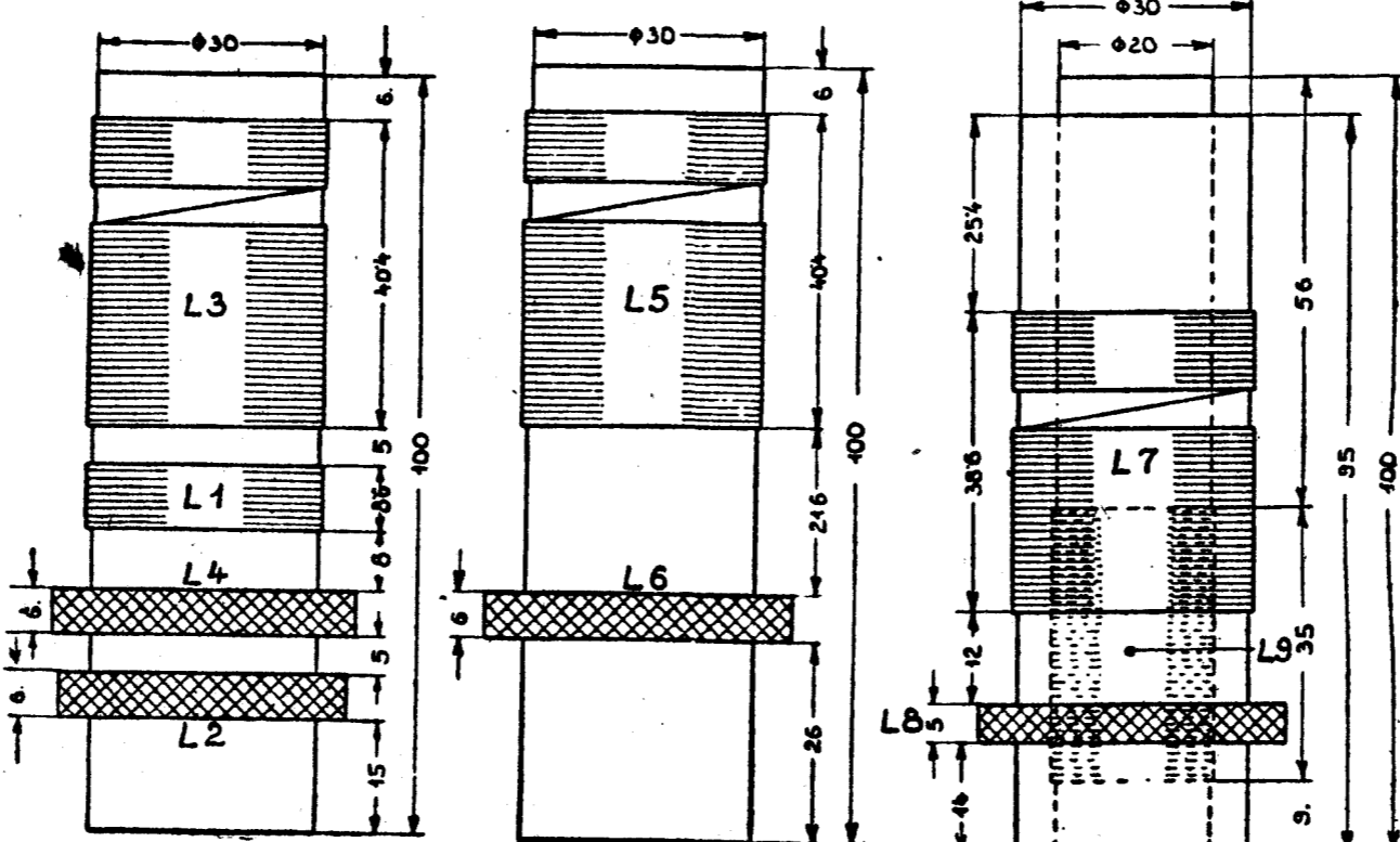
Detalles técnicos del esquema Tungram de cuatro válvulas
