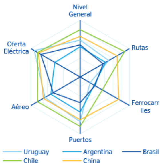
Gráfico 16. Calidad de las infraestructuras (año 2012)
